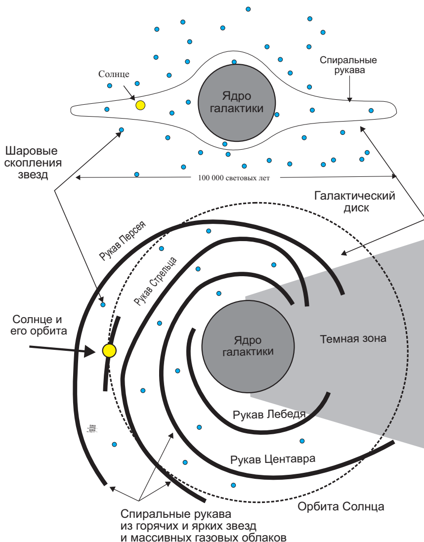
Рис. 2. Строение галактики Млечный Путь
