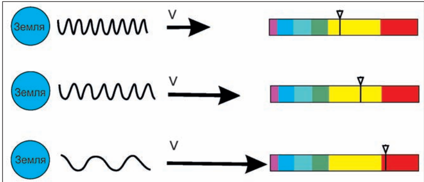
Рис. 3. Доказательство Большого взрыва. Все объекты Вселенной от нас удаляются. При удалении объекта смещение происходит в красную сторону спектра. Эффект Доплера (из кн.: Короновский, Брянцева, 2019)
