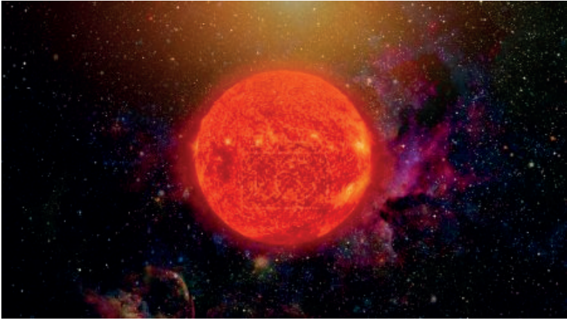
Рис. 5. Солнце – желтый карлик класса G2V ( https://photogenica.ru/preview-DP.php?directZoom=aVp1eDExSU04MUxNMG9HeVZ1eWpBZE9SY3BqalpxZFpTYzFWRjJ2dGZCcHJFbmZ6SVhIVDI1bTh3WWFPWkxneUhlMklydHQ0NjFITnZEL1BDU0pLOXlhTjY4Nkgrc2NOTGlvWVWk4L1lxNzJrRG0zVDA0aXRtUkVpWmhQMnRIRDhRSG5HRm04cW9JM0hMTU05ZzE0MXJBPT0=&hash=55562672b073c7b0b9452ef6b09ae445d4ad77bb85edef79eb2b5815b80fa0a1 )
