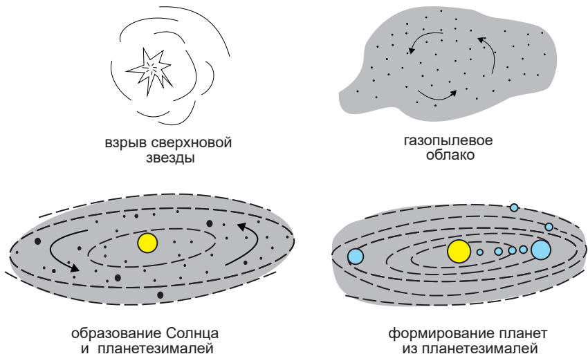
Рис. 4. Формирование Солнечной системы из газопылевого облака (из кн.: Короновский, Брянцева, 2019, упрощенно)
