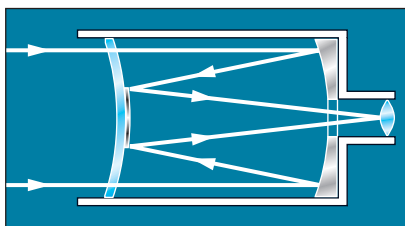
Рис. 1.5. Менисковый телескоп
