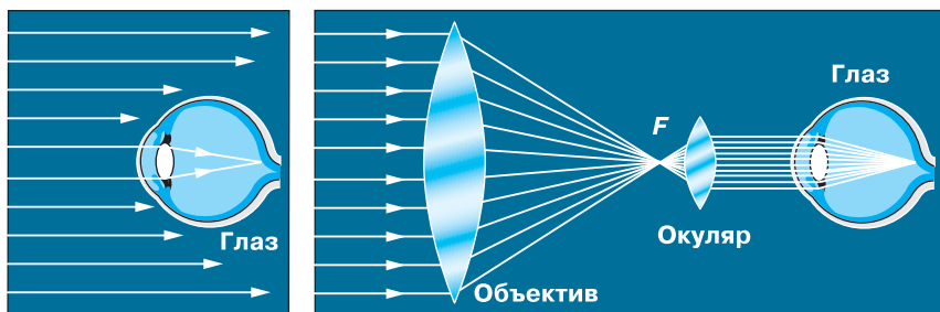
Рис. 1.4. Собираение света объективом телескопа
